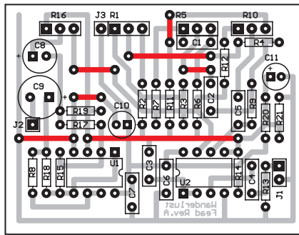
部品配置図
